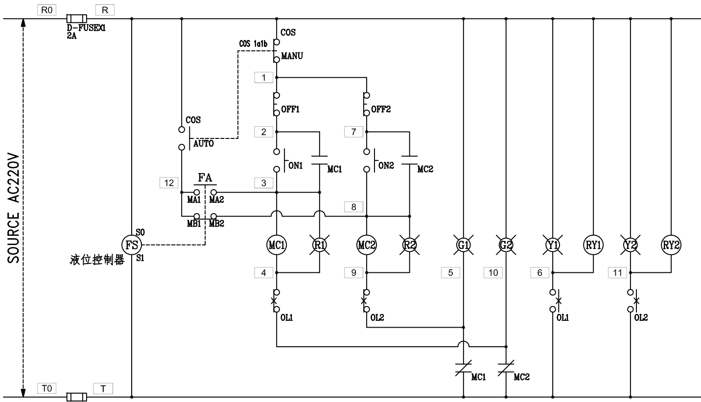
揚水泵交替運轉控制圖
