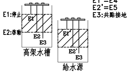
液位控制器 A-EF2 電極棒外接端子
