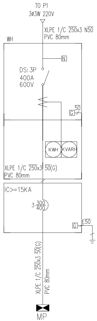
WH 結線圖 (不鏽鋼製)
