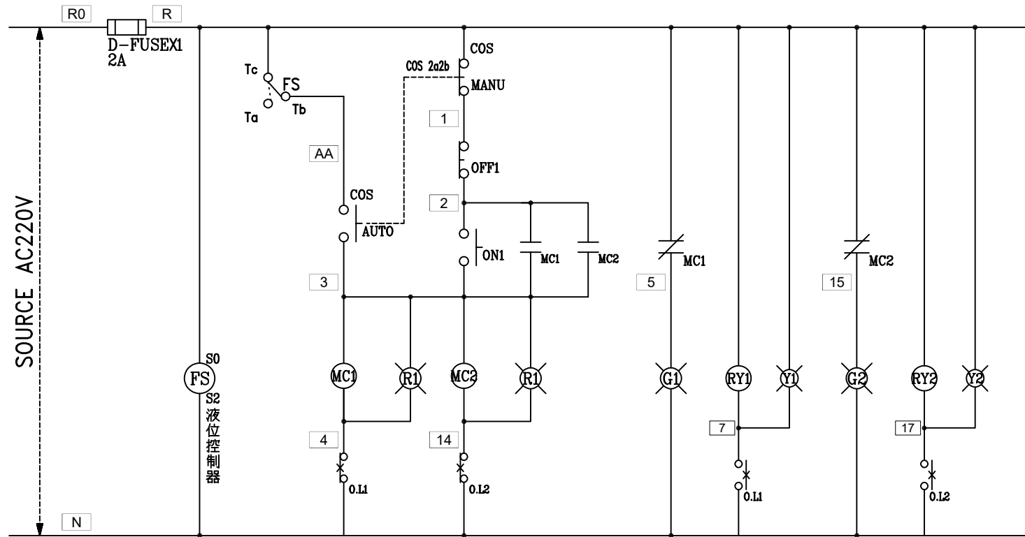
雨水回收池運轉控制圖
