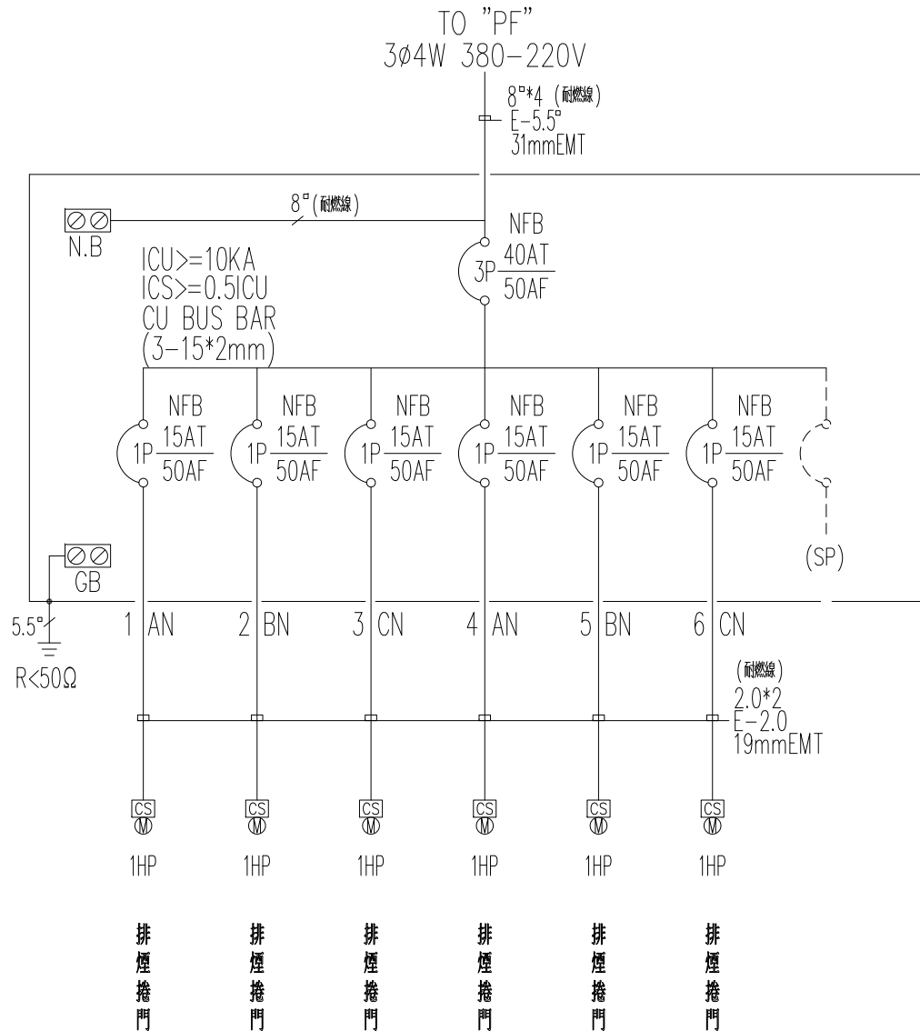
F1 PANEL LOAD: M=6HP
