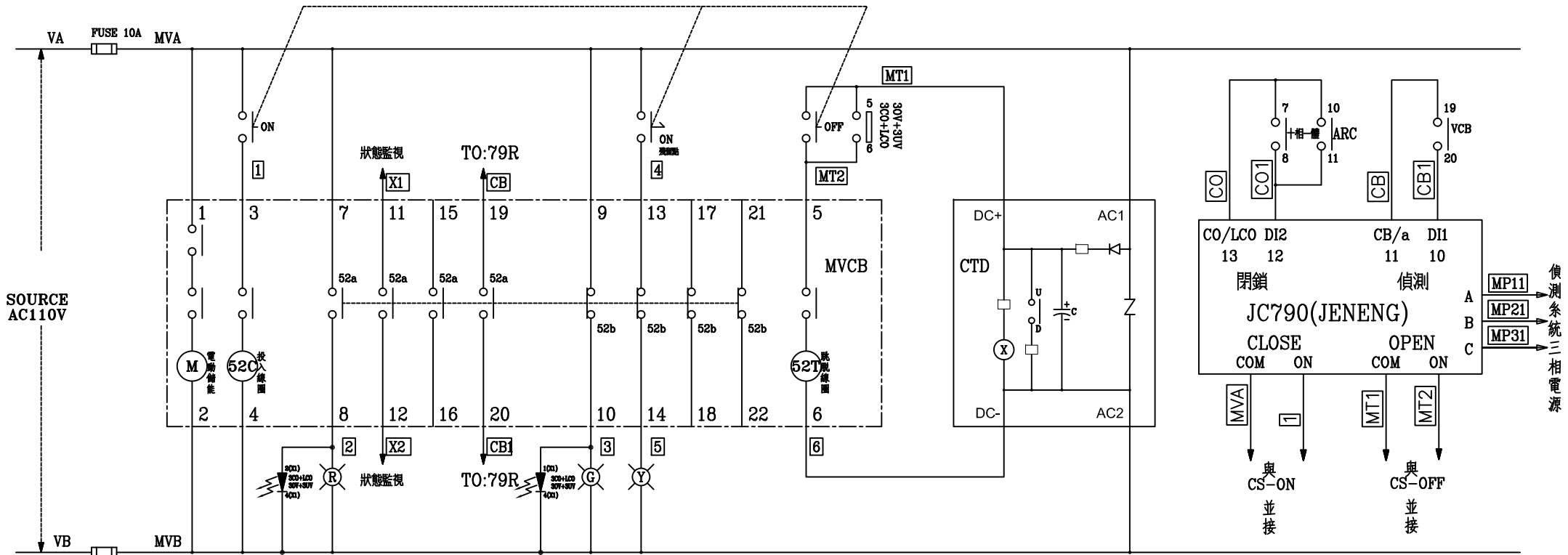
VCBA PANEL 20-VPR-16D MITSUBISHI "VCB" 控制圖
