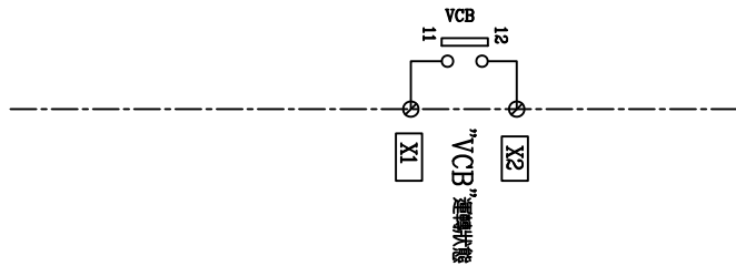
VCBA PANEL 20-VPR-16D MITSUBISHI "VCB" 控制圖
