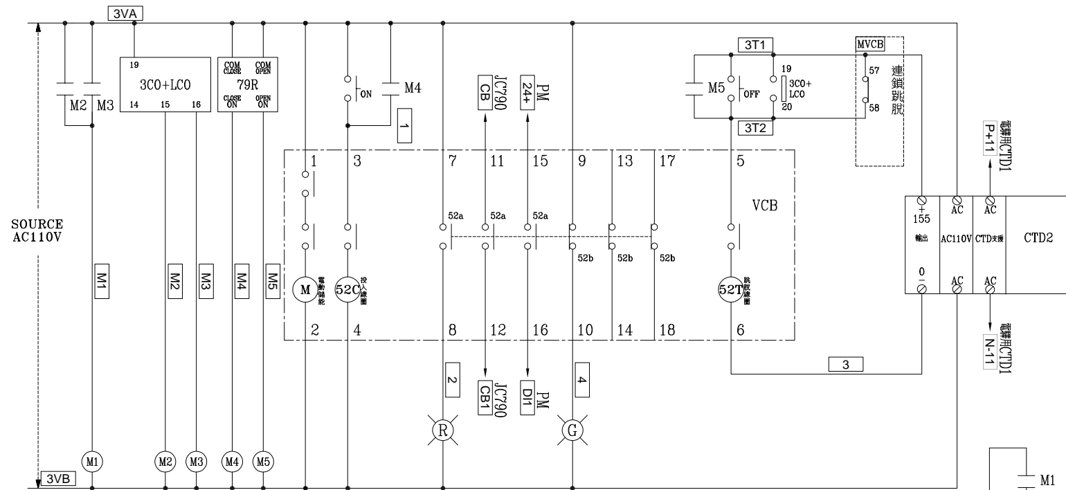
VCB3 PANEL MITSUBISHI "VCB" 控制圖
