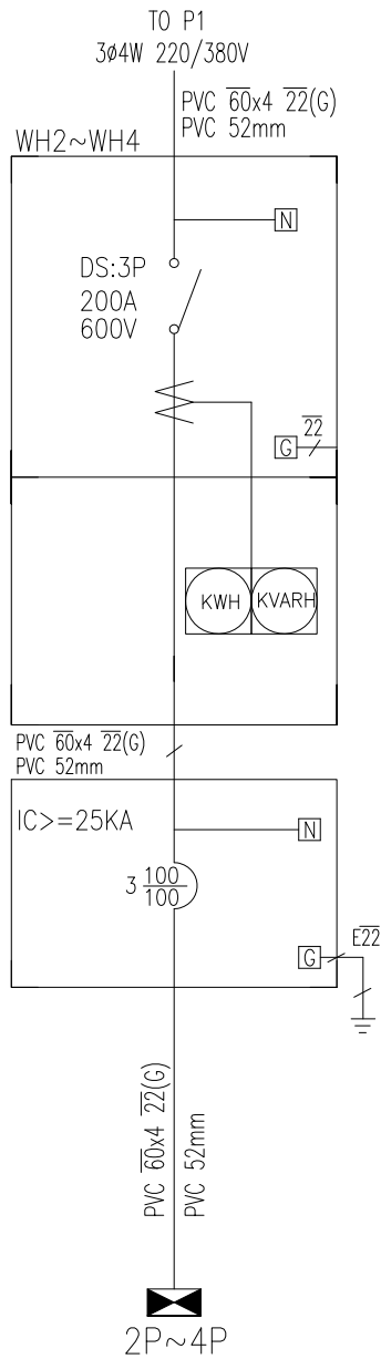
WH2~WH4 結線圖
