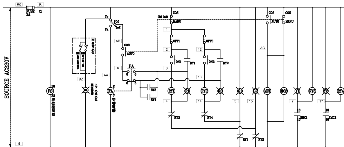
揚水泵交替運轉控制圖
