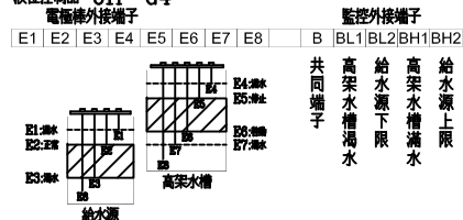
揚水泵交替運轉控制圖
