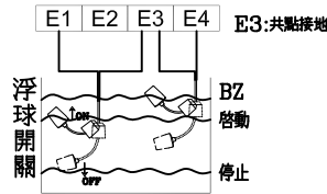
液位控制器 61F-G2 浮球外接端子
