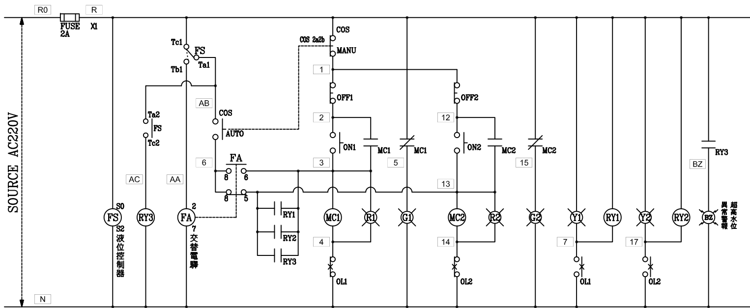
污.廢水泵(交替並列)運轉控制圖
